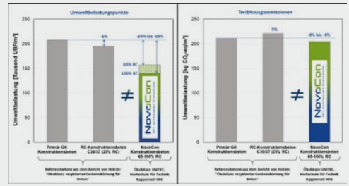
Abbildung 1: Resultat der Ökobilanz mittels UB-P-Methode für zwei Referenzbetone (Seite 1 und 2) und den NovoCon Konstruktionsbeton der Firma Möckli Beton AG (Seite 3). Der NovoCon Konstruktionsbeton spart rund 24% bis 33% jährlich vom RC-Gehalt zuzüglich 65% bis 100% der Umweltbelastung gegenüber einem Primärkonstruktionsbeton ein.
